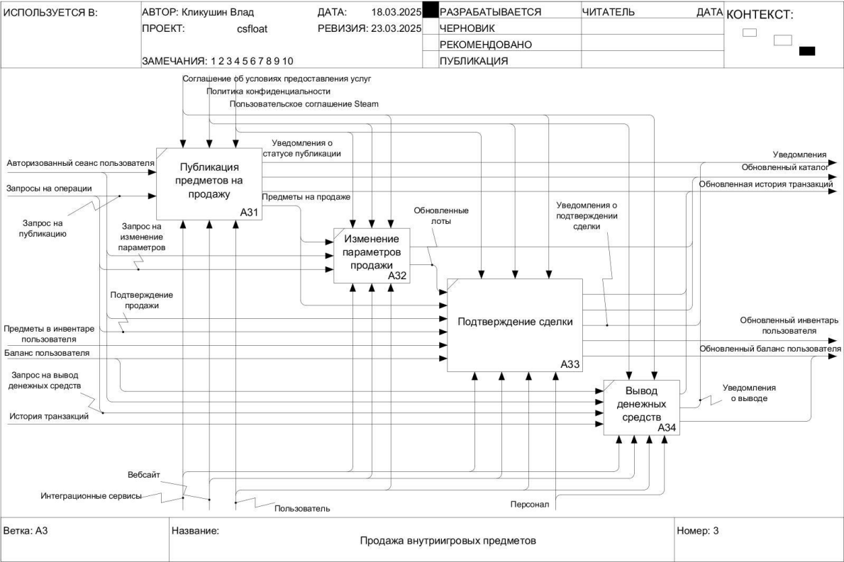
Рисунок 2.3.1 - Диаграмма декомпозиции процесса «Продажа внутриигровых предметов»
